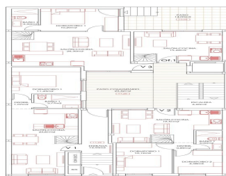
PLANTA BAJA, DESPUÉS DE LPO
