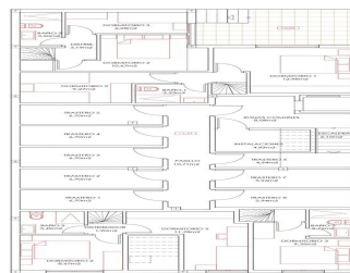
PLANTA SÓTANO, DESPUÉS DE LPO
