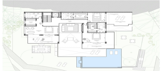
PLANTA ENTORNO
