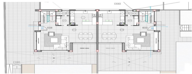
PLANTA BAIXA - SUPERFÍCIES SUP. CONSTRUÏDA TOTAL: 118,00m 2 (INCLÒSIVAS 18,00m 2 SOTERRAN) Casa Passeig de la Marina, 216 SUP. ÚTIL: 10,00m 2 (INCLÒSIVAS 18,00m 2 SOTERRAN) SUP. ÚTIL: 18,00m 2 Casa Carrer Estrella de Mar, 23 SUP. ÚTIL: 12,00m 2 (INCLÒSIVAS 18,00m 2 SOTERRAN) SUP. ÚTIL: 18,00m 2
