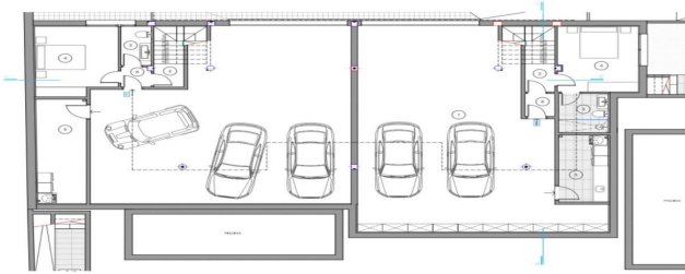
PLANTA SOTERRAN - SUPERFÍCIES SUP. CONSTRUÏDA TOTAL: 63,00m 2 Casa Passeig de la Marina, 216 SUP. ÚTIL: 18,00m 2 Casa Carrer Estrella de Mar, 23 SUP. ÚTIL: 12,00m 2
