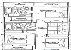
PLANTA ALTA SUPERFICIE ÚTIL CERRADA : 47.80m 2 SUPERFICIE CONSTRUIDA CERRADA : 60.87m 2 SUPERFICIE CONSTRUIDA TERRAZA (50m 2 ) : 5.78m 2 TOTAL SUPERFICIE CONSTRUIDA: 66.65m 2
