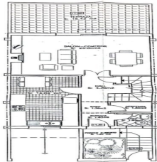
PLANTA BAJA SUPERFICIE ÚTIL CERRADA : 36.30m 2 SUPERFICIE CONSTRUIDA CERRADA : 60.87m 2
