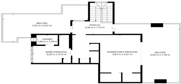
TOTAL: 160 m2 Planta baja: 106 m2, 1º piso: 54 m2 ÁREAS EXCLUIDAS: BALCÓN: 104 m2, MUROS: 15 m2
