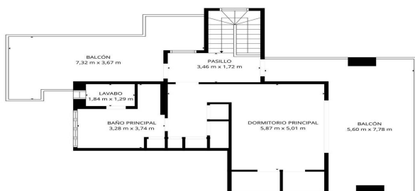
TOTAL: 160 m 2 Planta baja: 100 m 2 , 1 er piso: 54 m 2 ÁREAS EXCLUIDAS: BALCÓN: 104 m 2 , MUROS: 15 m 2
