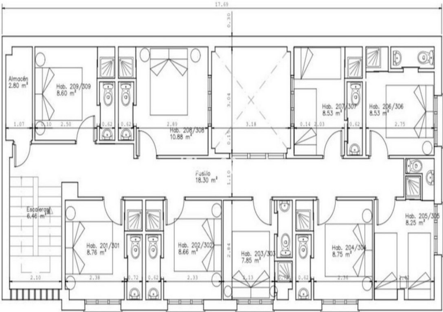
PLANTAS 2ª Y 3ª
