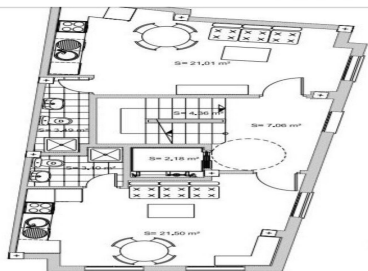
Plano Planta Primera
