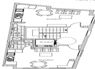
Plano Planta Segunda
