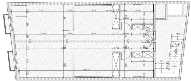
P2: Entrada &amp; Segundo Ascensor
